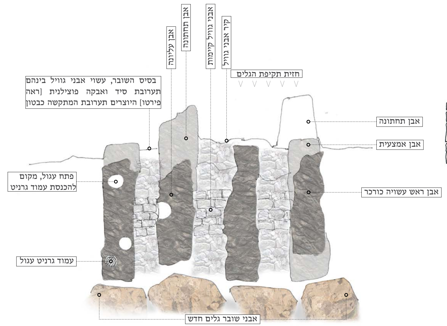
\\תכנית מצב קיים | שרידי שובר הגלים הדרומי
