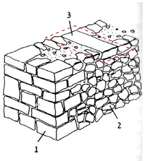
אופן בניית קירות אבן על פי ויטרוביוס 1. אופוס קוודרטום 2. אופוס אינקרטום 3. אבן קישור [ראש]
