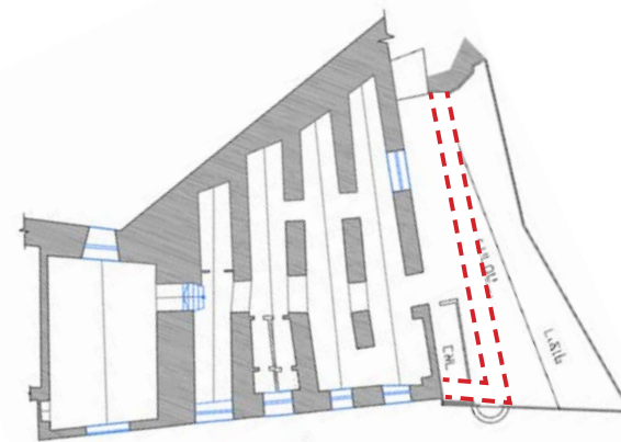
\\תכנית קומת קרקע עם מיקום משוער של קמרון נוסף שכיום הרוס מתוך תיק תיעוד קיר הים המזרחי
