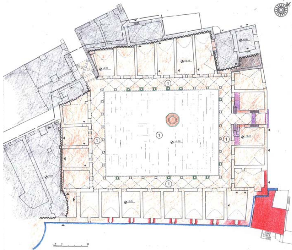
\\מפלס קרקע | מתוך סקר תיעוד חאן אל-עומדאן
