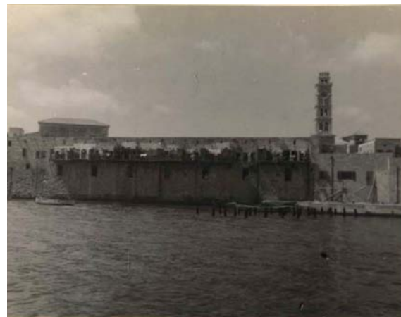
\תוספת מאוחרת של מרפסות אשר הוסרו בשנות ה-50. חזית הים מפלס עליון, מתוך דו"ח וינטר.
