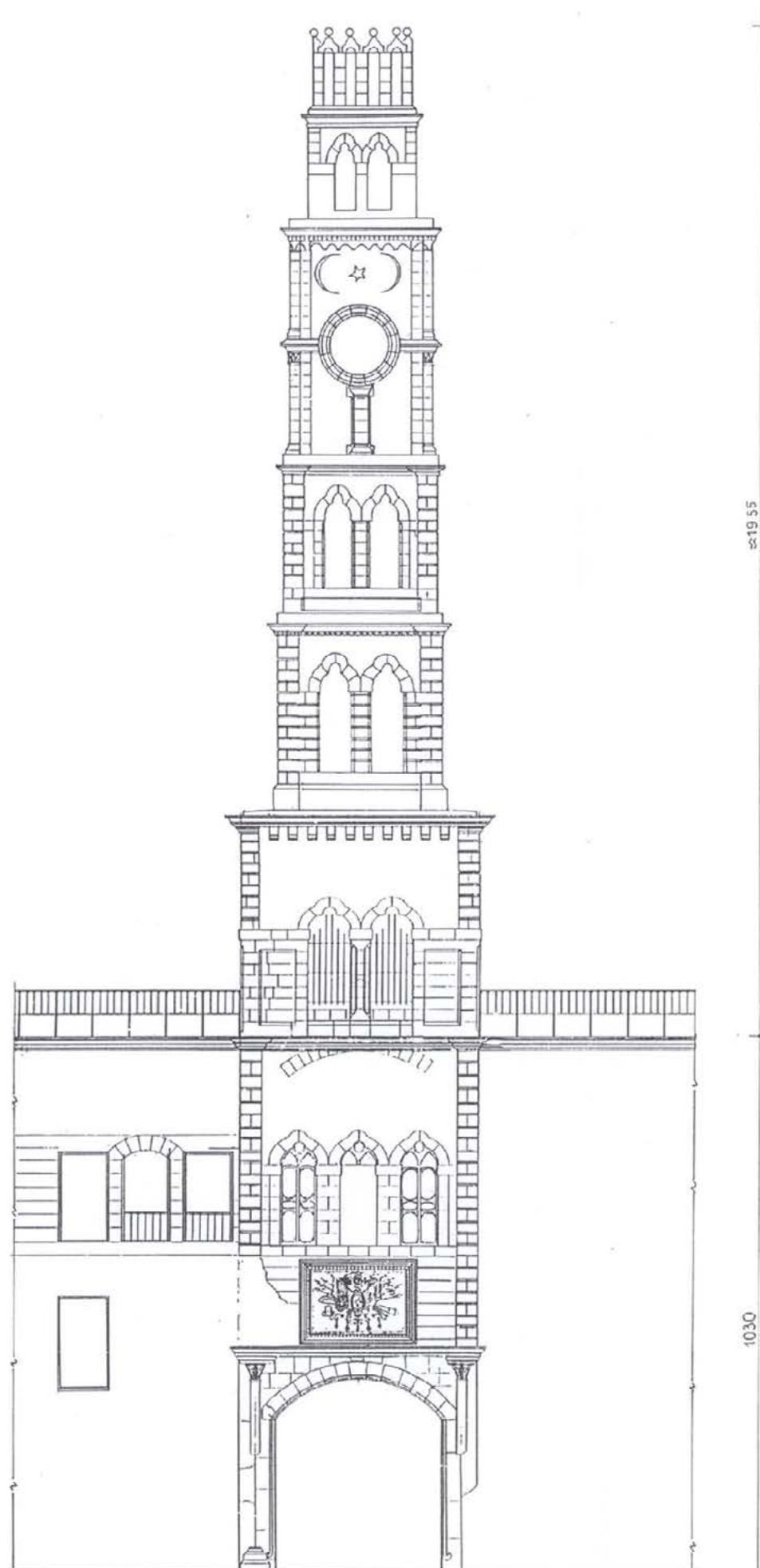
וורישום של חזית מגדל השעון ושער הכניסה לחאן אל-עומדן, מתוך סקר תיעוד החאן.
