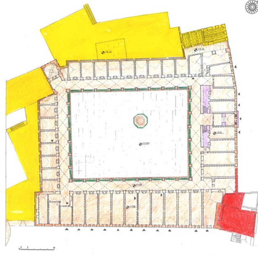
\\מפלס עליון | מתוך סקר תיעוד חאן אל-עומדאן
